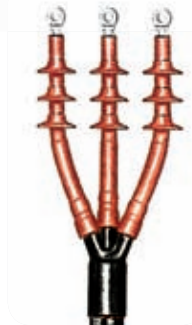
Dreipolige Endverschlüsse für Innen-/Außenanwendungen Für extrudiertes Kabel bis 36 Kv
