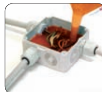
Verter Rayresin en la caja de empalme (1' máx.).
