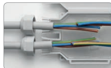
Moeren van tevoren aanbrengen en positionering van kabels
