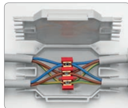
Verbinding van geleiders
