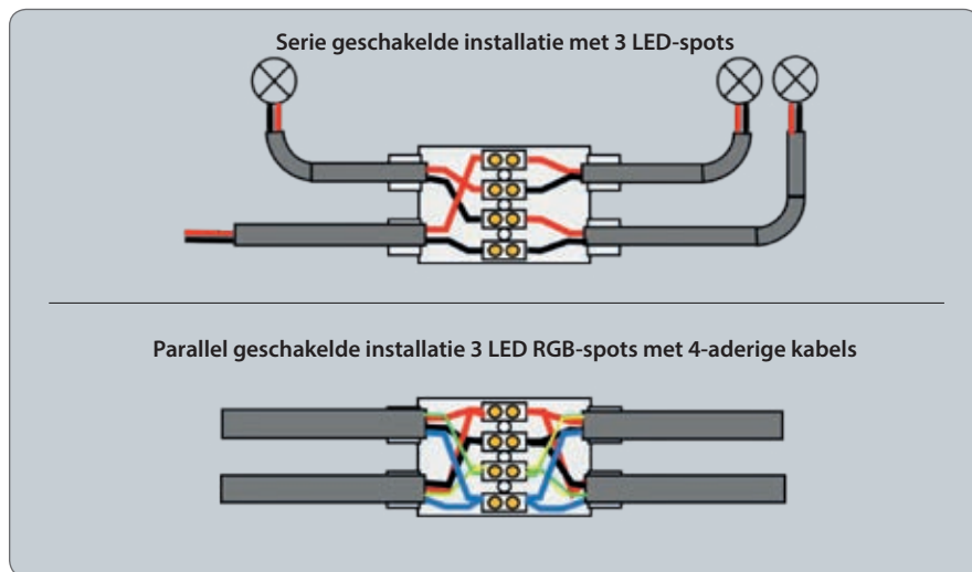
Verbinding van geleiders
