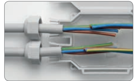
Pré-rosca e posicionamento de cabos
