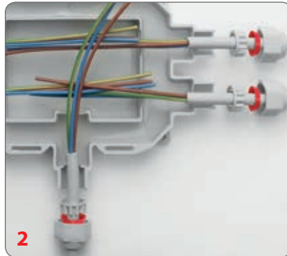
Porca e adaptador pré-rosçada e posicionamento de cabos.
