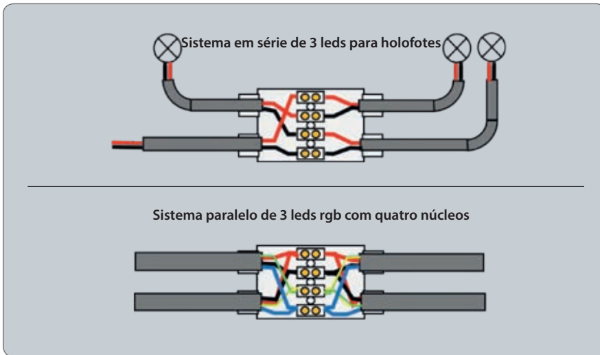
Conexão do condutor
