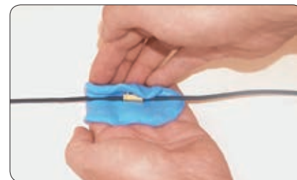
Isolamento de ligações múltiplas
