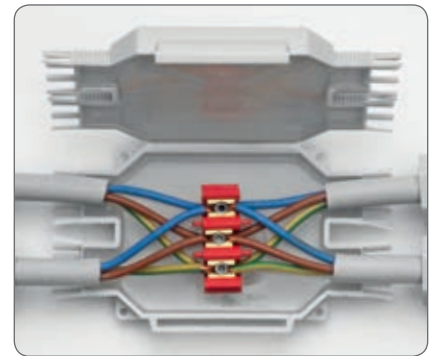
Conexão do condutor
