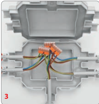
Conexão do condutor.
