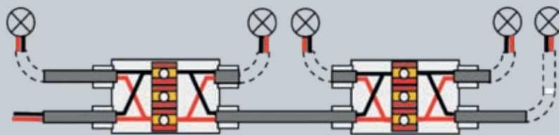
Installatie voor de parallele aansluiting van 5 lampen
